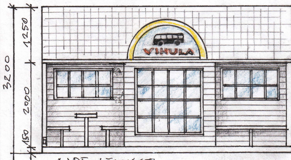
VAADE LÖUNAST
